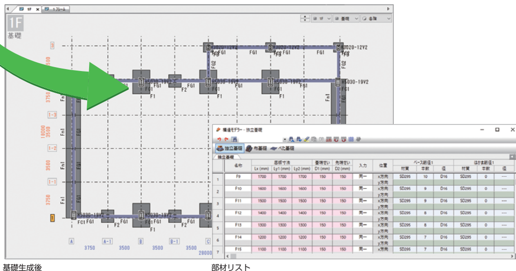
基礎生成後
