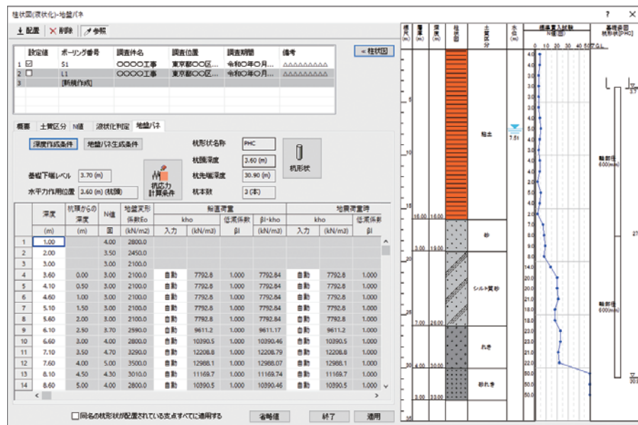
地盤バネダイアログ
