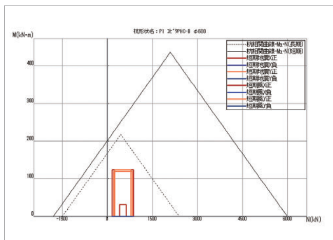
抗体M-N相關曲線図
