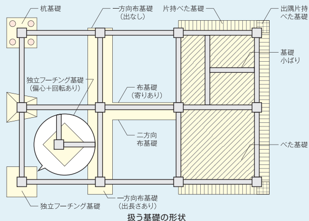
扱う基礎の形状
