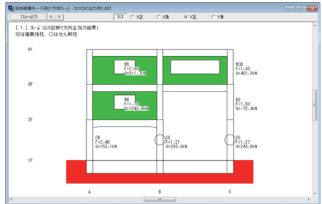
図17 診断破壊モード図(フレーム図)
